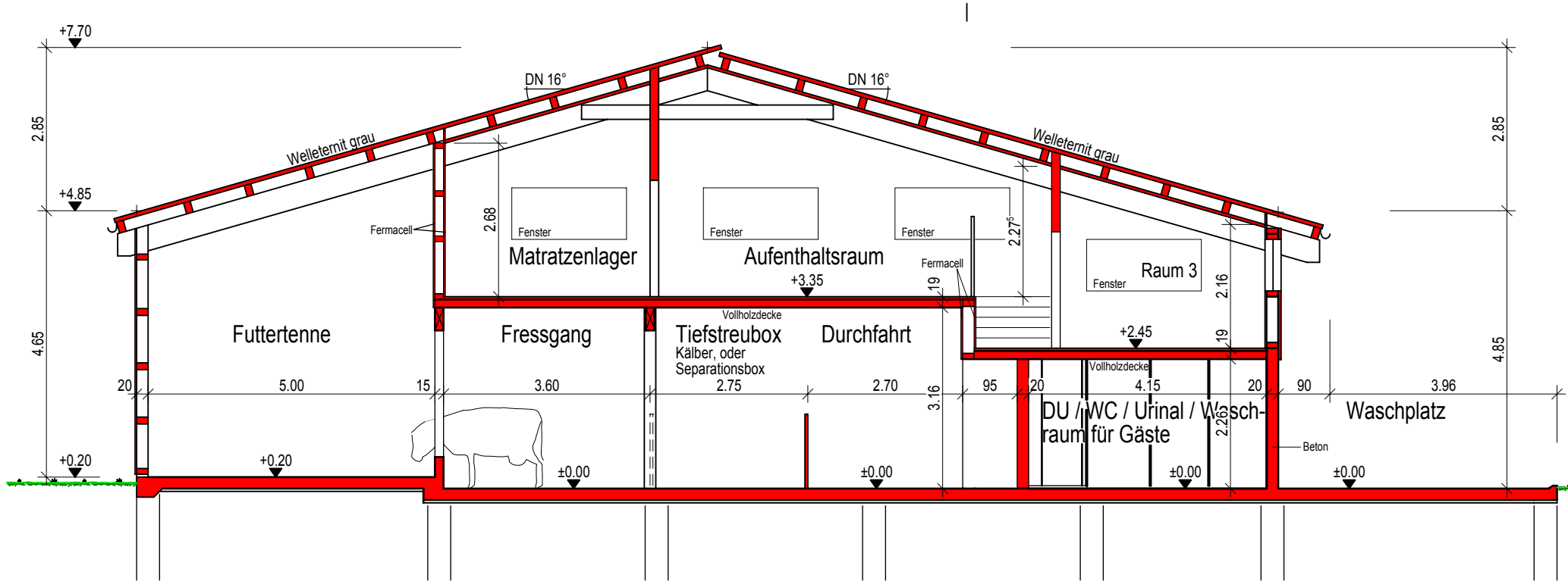
Schnitt A-A
